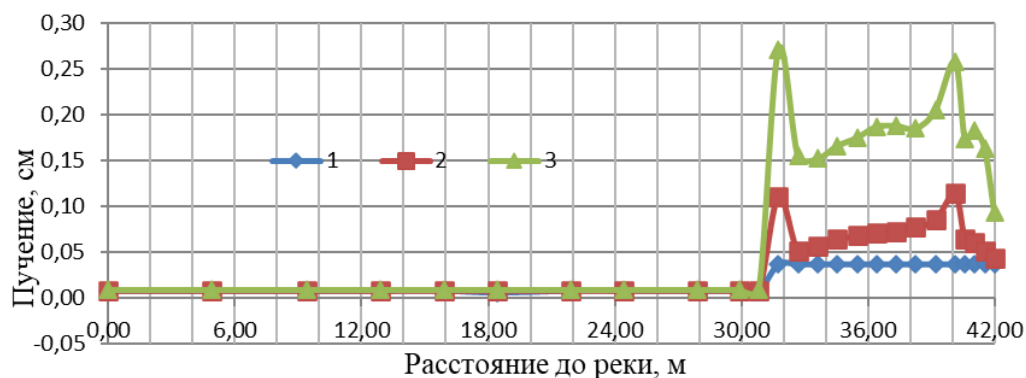
Рис. Динамика пучения грунта: 1 – начальное положение; 2 –сентябрь. 3 –апрель.
