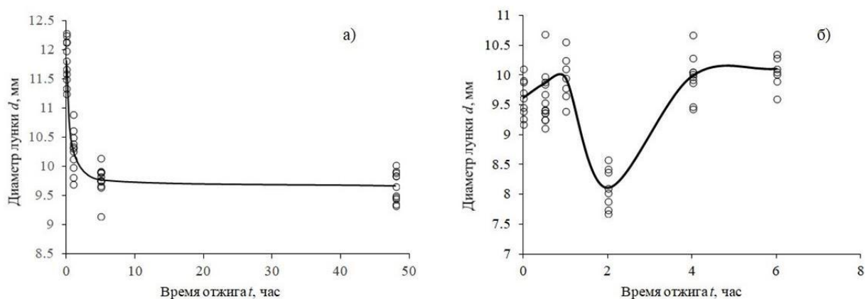
Рис. 2. Зависимость диаметра лунок d от времени отжига t . Температура отжига -1.5^{\circ}\text{C} (а), 0^{\circ}\text{C} (б). Температура проведения испытаний -12^{\circ}\text{C} .
