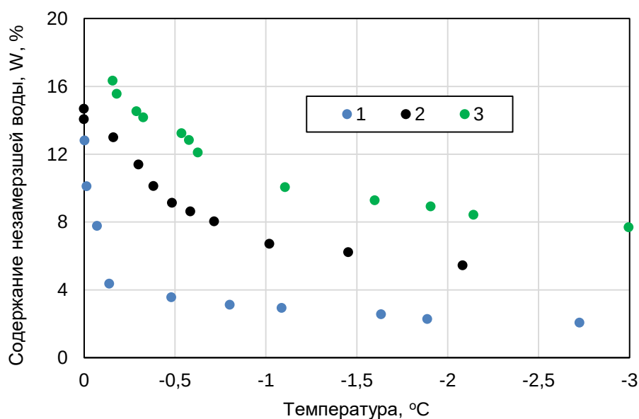
Рис. 1. Изменение содержания незамерзшей воды в области высоких отрицательных температур (до -3^{\circ}\text{C} ) в супесчано-суглинистых грунтах (г. Салехард) с различным содержанием органического вещества ( I_r ): 1- 0,94%, 2 – 1,76%, 3 – 5,51%.
