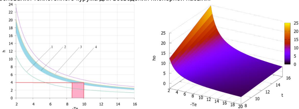
Рис. Изменение необходимой высоты техногенного курума для создания барьерного целика в зависимости от средней температуры пород деятельного слоя в конце периода проморозки при разной температуре воздуха в теплый период года: 1 – t = +7,0^{\circ}\text{C} ; 2 – t = +10,8^{\circ}\text{C} ; 3 – t = +12,8^{\circ}\text{C} ; 4 – t = +15,0^{\circ}\text{C}
