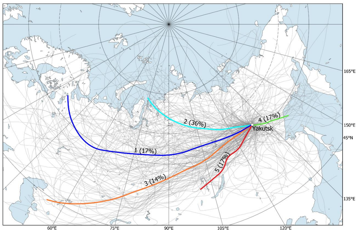
Рис. 2 Схема распределения источников влаги в атмосферных осадках на примере г. Якутска в период сентябрь 2017 г. - февраль 2024 г.
