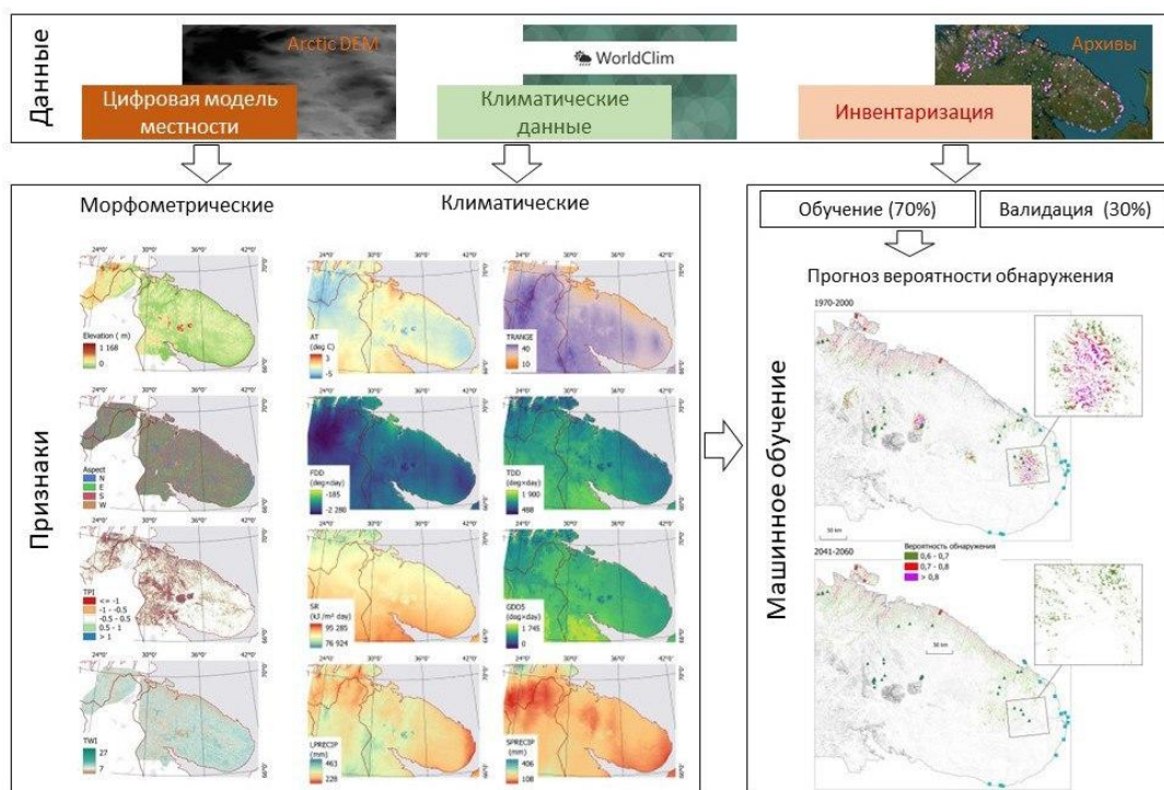
Рис. 1. Алгоритм прогнозирования распространения и динамики бугристых болот на Кольском полуострове.
