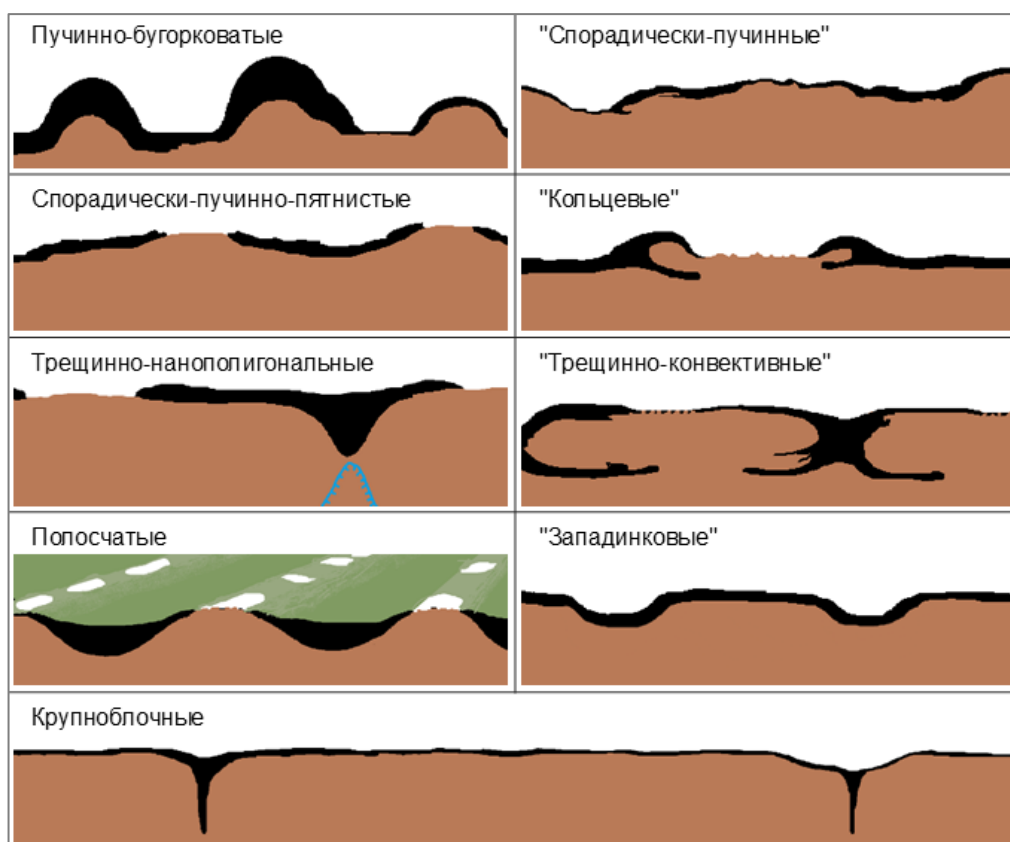
Рисунок 1. Типы криогенных микроструктур почвенного покрова, описанные автором в подзоне типичных тундр ЕТР. Черным цветом показаны органические горизонты почв, коричневым – минеральные. Названия даны в соответствии с Атласом Арктики (1985).
