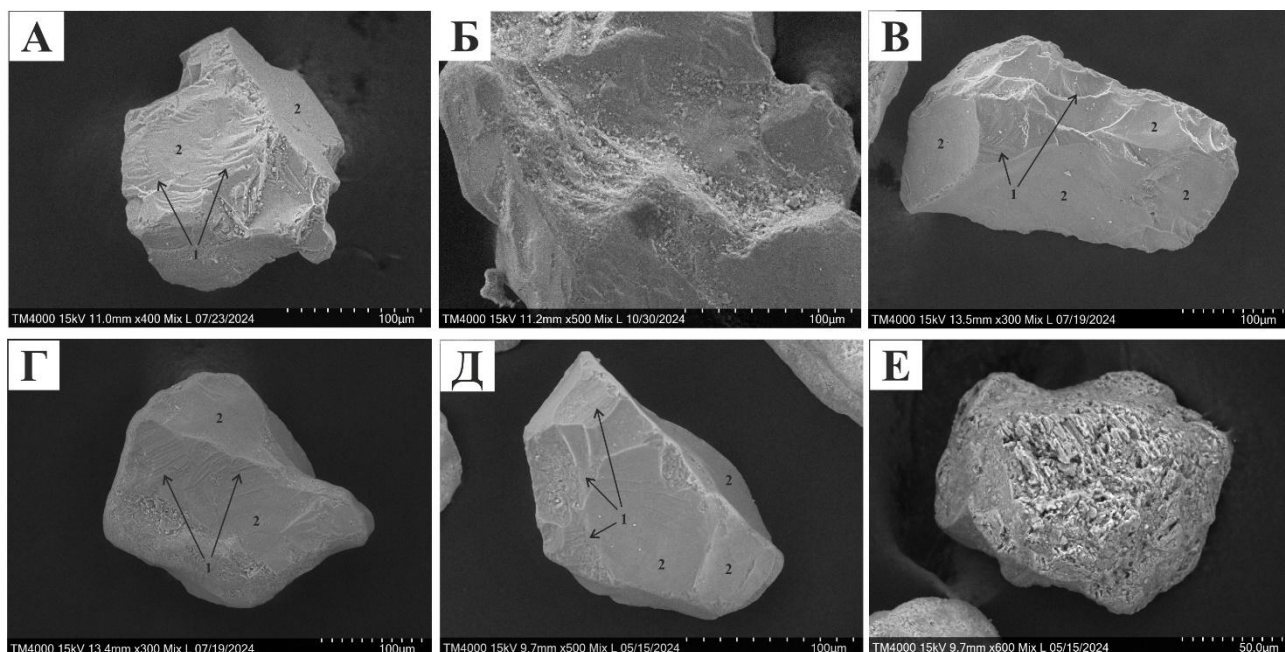
Рис. 1. Криогенный микрорельеф песчаных зёрен кварца: 1 – раковистые сколы, 2 – гладкие полированные поверхности (А – песчаное зерно из водноосадочных отложений; Б – увеличенный фрагмент раковистых сколов (водноосадочные отложения); В, Г, Д, Е – песчаные зёрна из субаэральные отложений).
