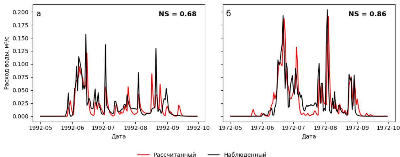
Рис. 1. Сравнение рассчитанных и наблюдаемых суточных гидрографов стока за 1992 (а) и 1972 (б) годы. Значения критерия Нэша-Сатклиффа (NS) указаны на графиках.
