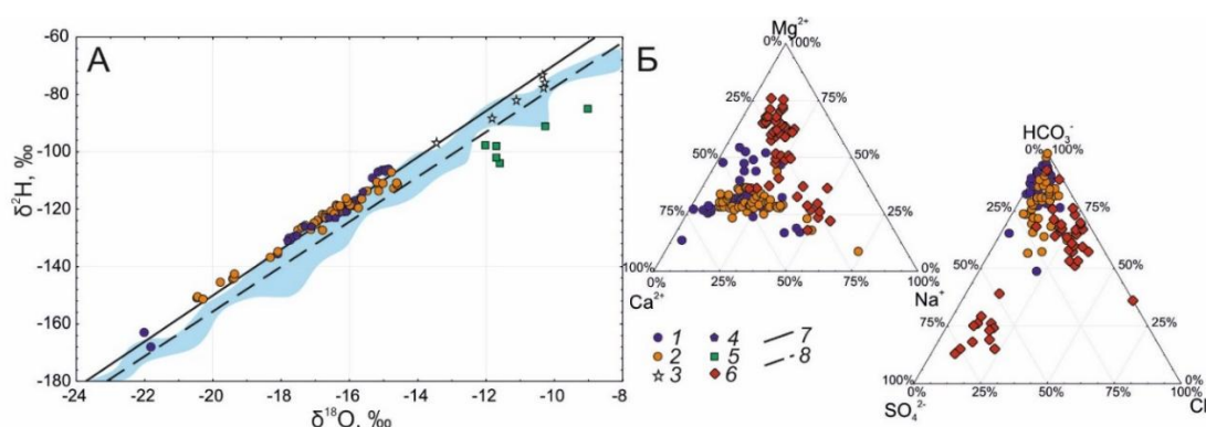
Рис.1. Изотопный (А) и макрокомпонентный (Б) составы природных вод г. Салехард: 1 – подземные воды 2024 г., 2 – поверхностные воды (лето 2023–2024 г.), 3 – дождь (август 2024 г.), 4 – подземные воды 2021 г. (Токарев и др., 2024), 5 – озера (2021, 2024 г.), 6 – поверхностные воды (2002 г.), 7 – глобальная линия метеорных вод (ГЛМВ), 8 – локальная линия метеорных вод (ЛЛМВ) в г. Салехард в 1996–2000 г ( https://nucleus.iaea.org/wiser/explore ), на врезке заливкой показана область изотопного состава атмосферных осадков г. Салехард
