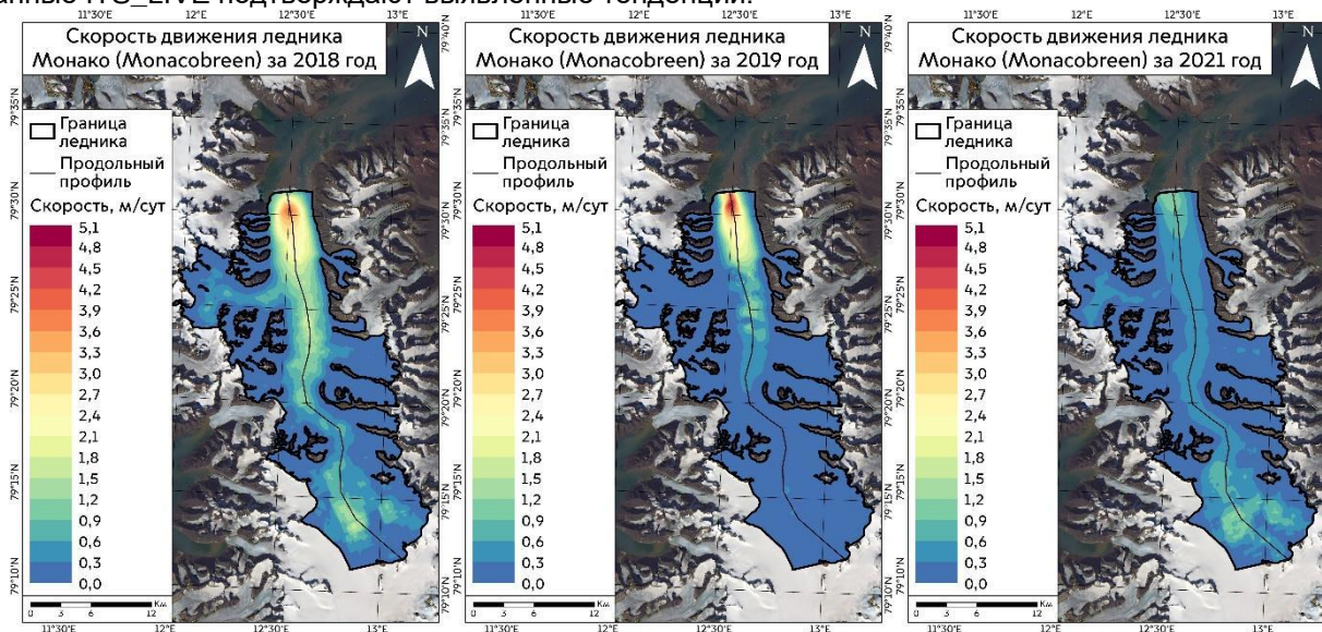
Рис. 4. Среднегодовая скорость движения ледника Монако за 2018 год (слева), 2019 год (в центре) и 2021 год (справа), составлено автором.
