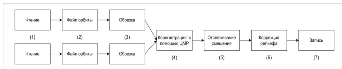
Рис. 1. Процесс обработки снимков в ПО SNAP для получения скоростей движения ледников, составлено автором.
