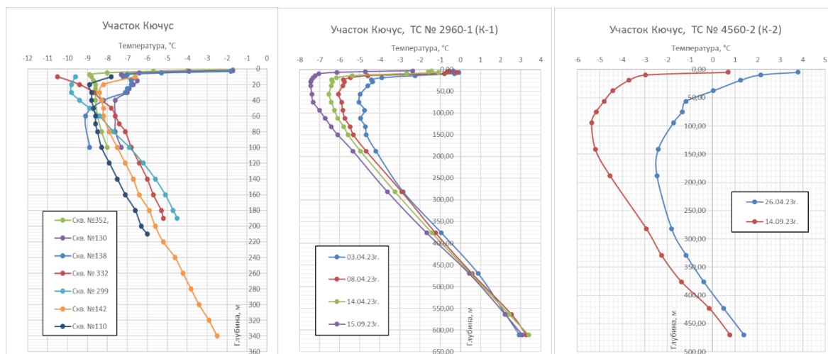
Рис. 1. График изменения температуры горных пород участка Кючус.
