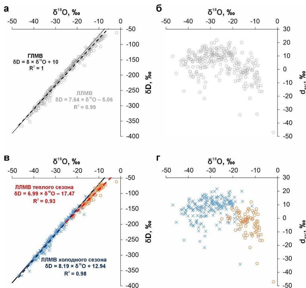
Рис. 1. Изотопный состав атмосферных осадков г. Якутска: а) \delta^{18}\text{O}/\delta\text{D} , б) \delta^{18}\text{O}/d_{\text{exs}} , в) \delta^{18}\text{O}/\delta\text{D} по сезонам, г) \delta^{18}\text{O}/d_{\text{exs}} по сезонам.
