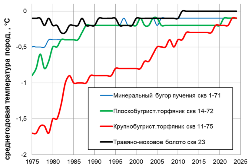
Рисунок. Изменение среднегодовой температуры многолетнемерзлых пород
