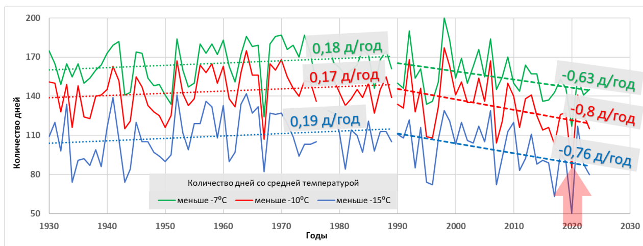
Рис. 1 Количество дней со средненежной температурой меньше -7°C (зелёная), -10°C (красная) и -15°C (синяя кривая) по данным метеостанции Салехард.
