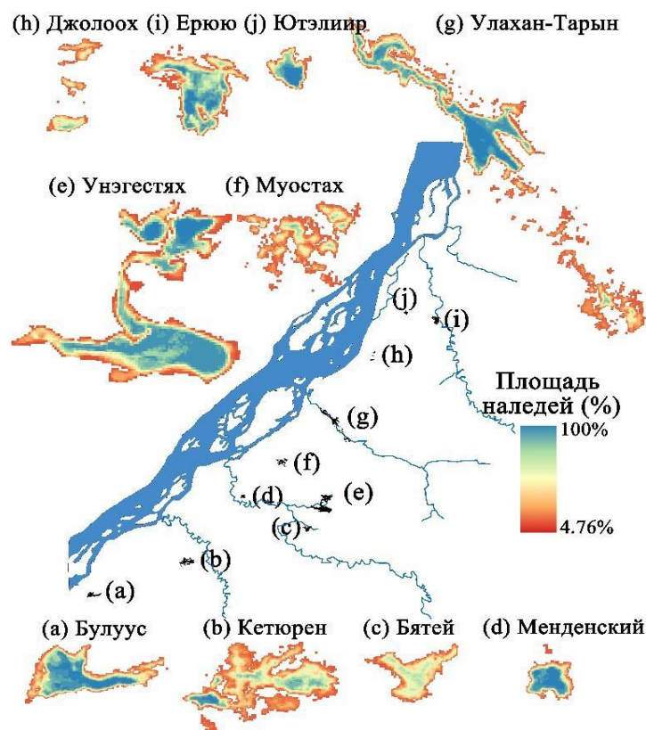
Рис. 1. Вероятность покрытия поверхности земли наледями в Центральной Якутии в 2002-2022 гг.
