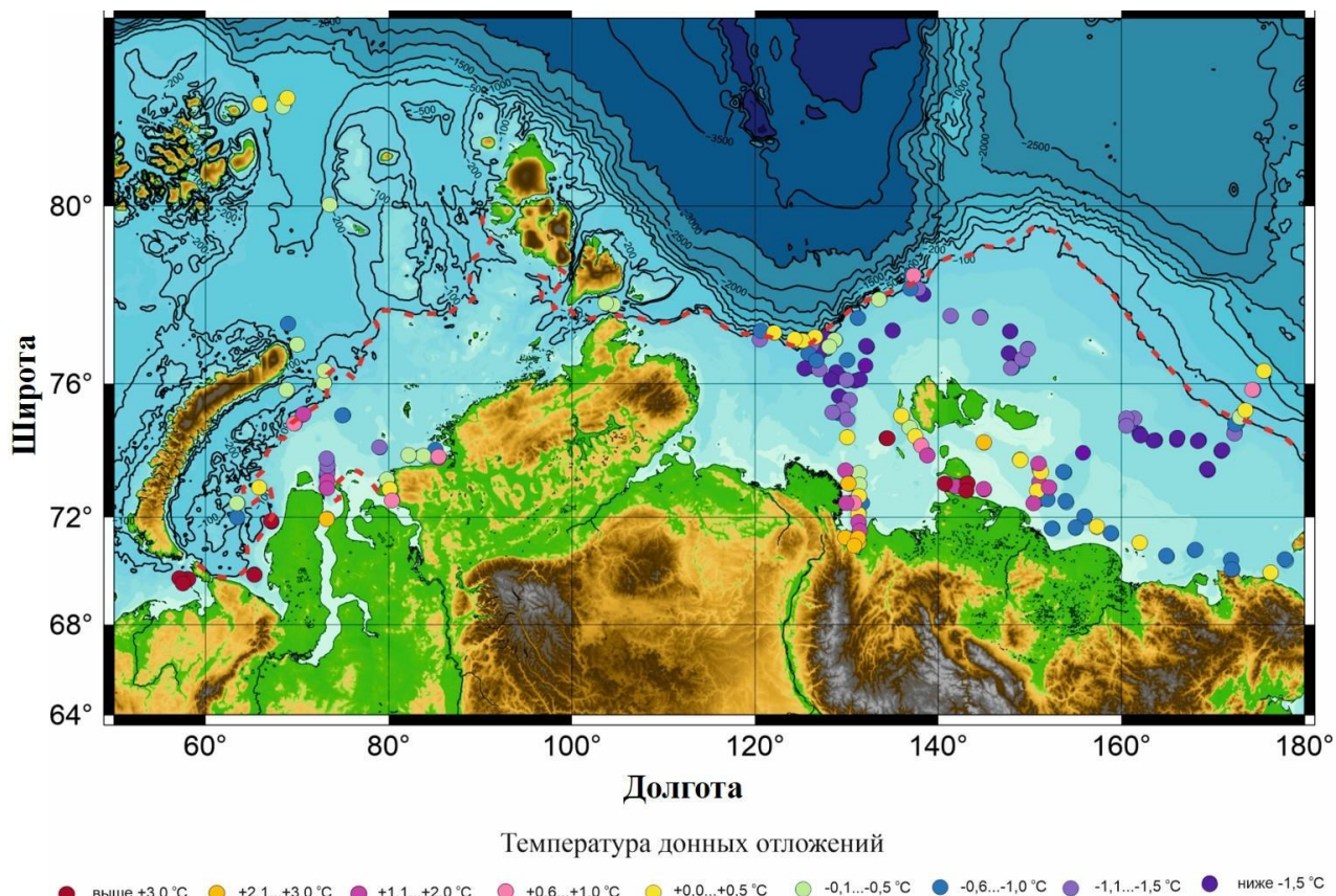
Рис. 1. Распространение температуры донных отложений арктических морей РФ (по данным https://doi.org/10.1016/j.marpetgeo.2023.106467 ).
