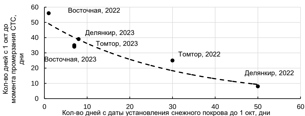
Рис. 1. Зависимость срока промерзания СТС от момента установления снежного покрова для Верхоянского региона.
