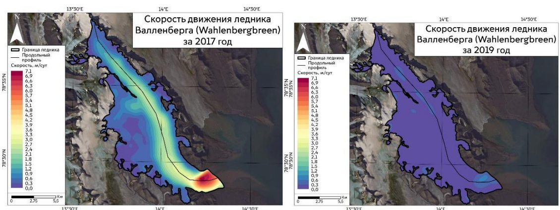
Рис. 2. Среднегодовая скорость движения ледника Валленберга за 2017 год (слева) и 2019 год (справа), составлено автором.
