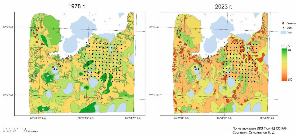
Рис. 1. Глубина сезонного протаивания в урочищах геокриологического стационара Марре-Сале в 1978 и 2023 гг.
