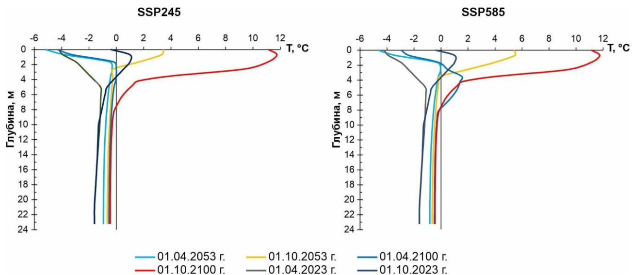
Рис. 1. Результаты моделирования температурного режима пород.
