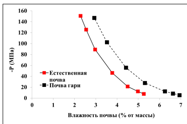
Рис. 2. Зависимость потенциала влаги от влажности в слое почвы 5-30 см в диапазоне пленочной влаги
