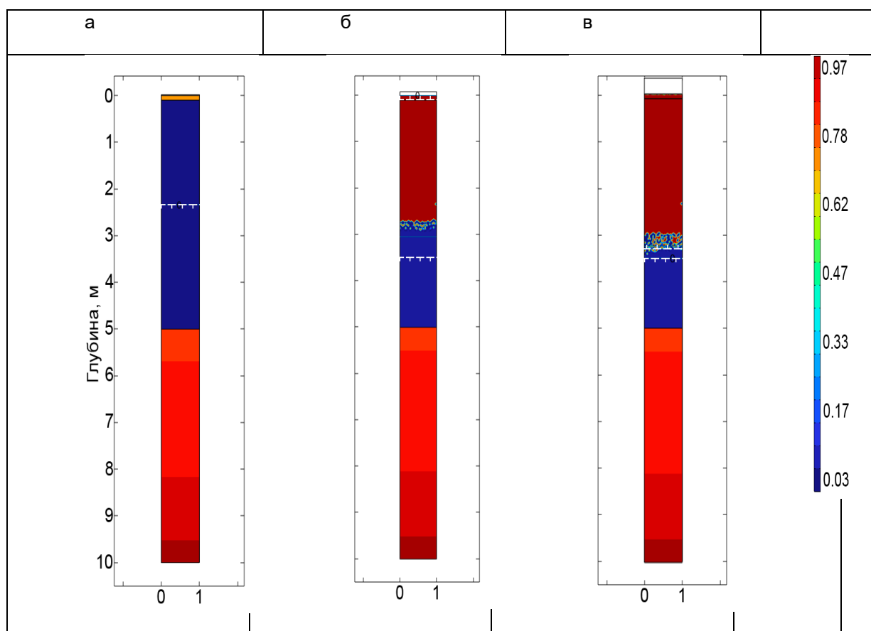
Рис. 1. Изменение заполнения пор влагой деятельного слоя: а – при нулевой начальной влажности (начало расчета, 1 сентября); б – на 30 день с начала расчетов; в – на 145 день с начала расчета (конец января)
