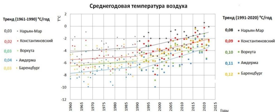
Рис. 1. Тренды среднегодовой температуры воздуха на метеостанциях Европейского севера
