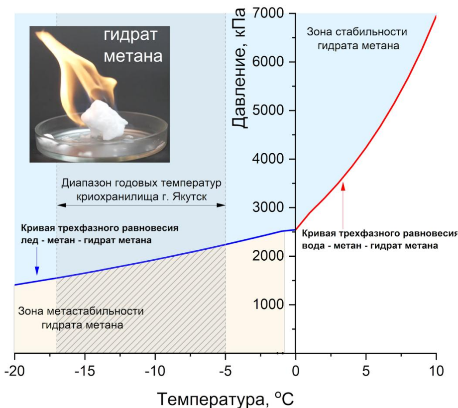
Рис. 1. Зоны существования гидратов метана в стабильном и метастабильном состоянии.
