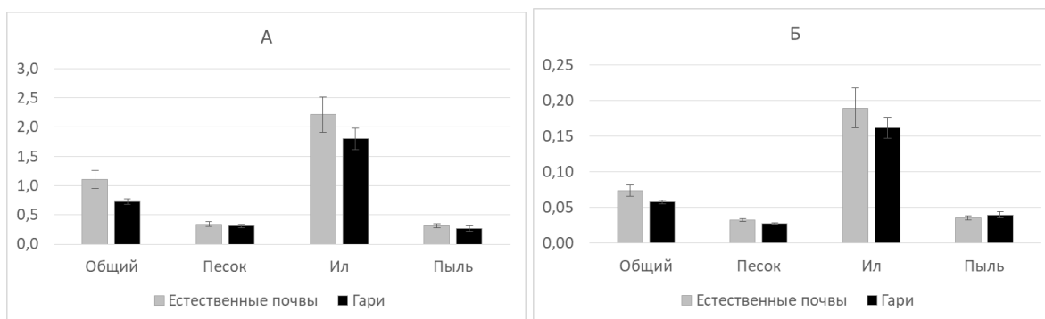
Рис. 1. Содержание общего углерода (А, %) и азота (Б, %) в слое 5-30 см (общий) и в гранулометрических фракциях (песок, пыль, ил) почвы гари и ее естественного аналога
