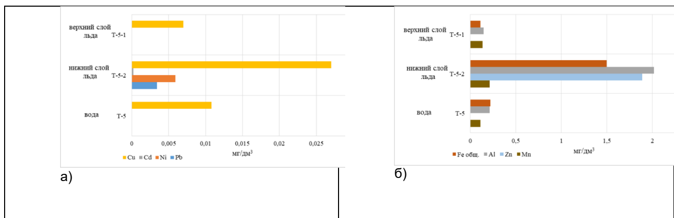
Рис. 2. Динамика изменения некоторых микроэлементов в верхних и нижних толщах льда
