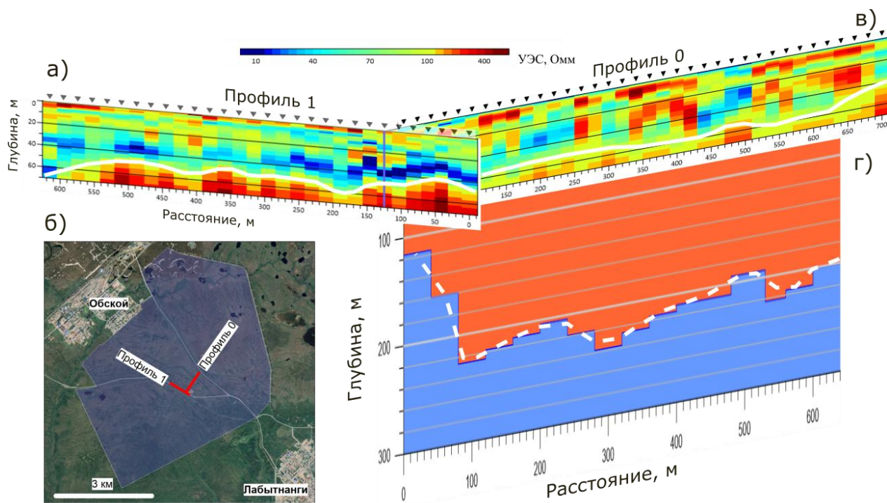
Рис. 1. а) геоэлектрический разрез по профилю 1 по результатам зондирований методом РМТ-К; б) схема полигона «Семь лиственниц» с обозначенными профилями геофизических работ; в) геоэлектрический разрез по профилю 0 по результатам зондирований методом РМТ-К; г) изменение глубины проводящего основания (синий цвет) вдоль профиля 0 по результатам зондирований МПП. Сплошной белой линией обозначена предполагаемая кровля (а, в), пунктирной белой линией – подошва реликтовой мёрзлой толщи (г).
