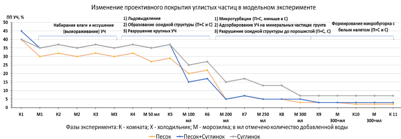
Рис. 2. Динамика ПП УЧ в зависимости от количества циклов промораживания-протаивания и количества добавленной воды
