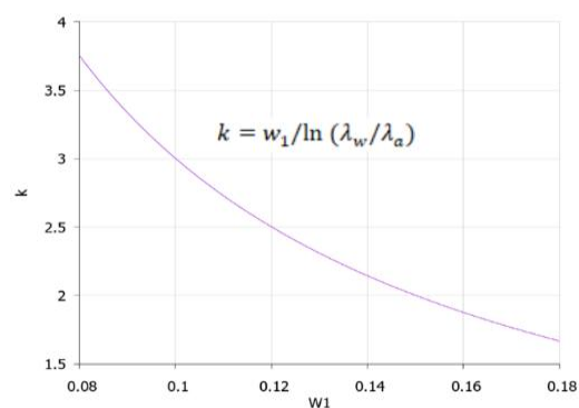
Рис.2. А) - степень изменения глубины оттаивания « \mu » на второй год после снежной мелиорации в зависимости от начальной влажности грунта « W_1 » (до проведения снежной мелиорации): 1 - W_1 = 0,1 ; 2 - W_1 = 0,12 ; 3 - W_1 = 0,14 . 4 - W_1 = 0,16 ; Б) - оптимальное значение степени увлажнения грунта деятельного слоя « k » для достижения максимального уровня снижения глубины оттаивания « \mu » на второй год.
