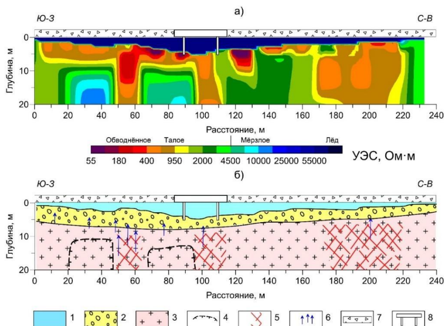
Рис. 1 Геоэлектрический разрез по профилю по данным БИЭП (а) и его интерпретация (б): 1- лёд; 2 – рыхлые отложения; 3 – гранитоиды; 4 – граница ММП; 5 – зоны дробления; 6 – каналы фильтрации подземных вод; 7 – дорожное полотно; 8 – мост.
