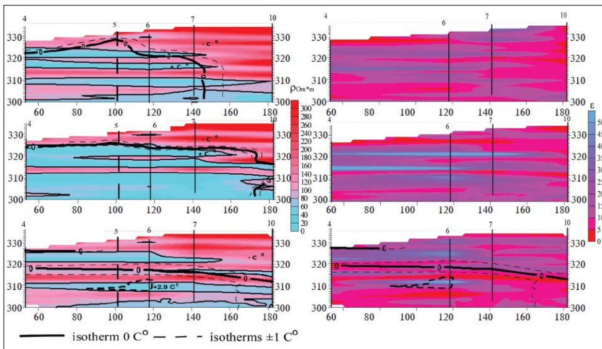
Рис.1. Примеры геоэлектрических разрезов: слева – эффективных сопротивлений ( \rho ); справа – относительной диэлектрической проницаемости ( \epsilon ), по профилю скважин (4–5–6–7–10) в мерзлом массиве вкост береговой линии Сытыканского гидроузла (Зап. Якутия); наблюдения ДИМЧ: сверху – март 2001; в середине – август 2001; внизу – март 2002. Для мерзлых пород характерно высокое \rho и низкое \epsilon ; для талых – низкое \rho и высокое \epsilon . Уровень дна около плотины 301 м. По горизонтальным осям расстояние от береговой линии, по вертикальным – абсолютные отметки глубины, [м].
