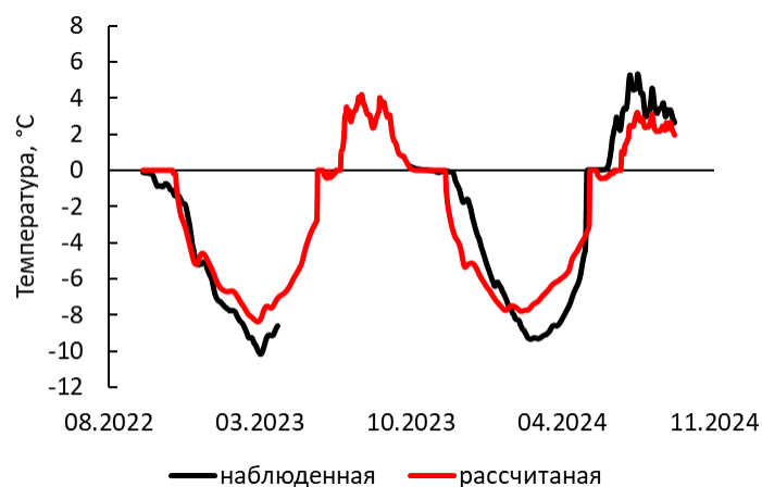
Рис. 2. Сравнение рассчитанных и наблюдаемых температур пород на глубине 1 м.
