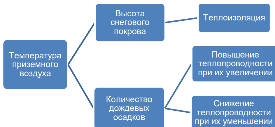
Рис. 1. Схема взаимосвязи климатических факторов с типом их воздействия на тепловой поток, изменяющий состояние грунтов.
