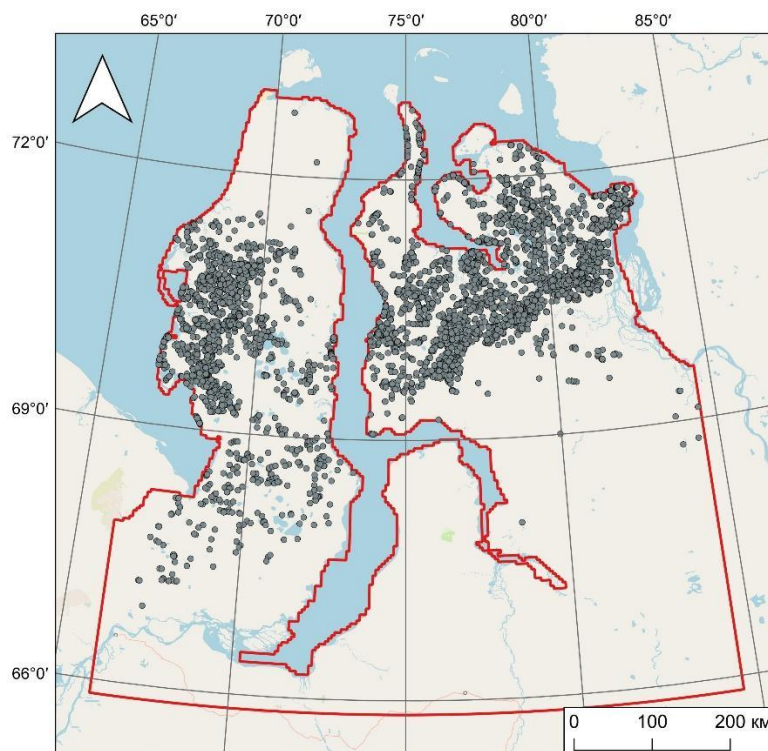
Рис. 1. Идентифицированные ТФР на севере Западной Сибири (подложка OpenStreetMap).
