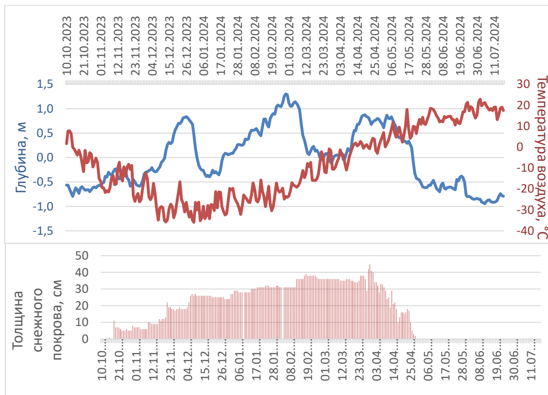
Рис. 2. Графики сопоставления уровней подземных вод в скважине №1-23, температуры воздуха (верхний) и толщины снежного покрова (нижний) по данным метеостанции в г. Тынды
