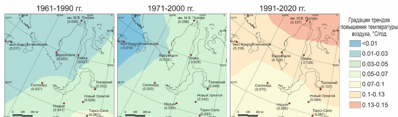
Рис. 1. Карты-схемы пространственного изменения трендов среднегодовой температуры воздуха западного сектора Российской Арктики.
