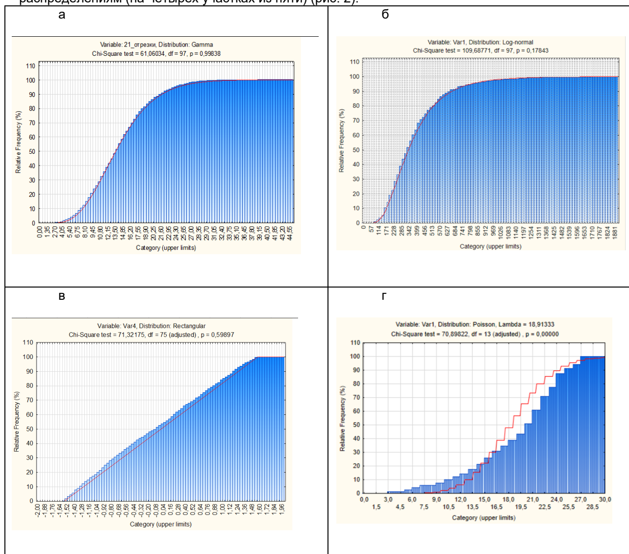
Рис. 2. Пример степени соответствия теоретических и эмпирических распределений для 21 участка: а) длины отрезков (гамма-распределение), б) площади полигонов (логнормальное распределение), в) углы отрезков (равномерное распределение), г) число центров полигонов на случайно выбранной площадке (распределение Пуассона); синий контур – эмпирическое распределение, красная линия – теоретическое распределение.
