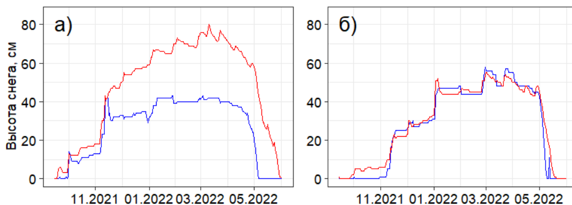
Рис. 2. Сравнение наблюдаемой высоты снега с высотой снега по данным ERA5-Land для станций Сусуман (а) и Коркодон (б).
