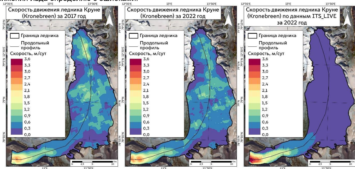
Рис. 3. Среднегодовая скорость движения ледника Круне за 2017 год (слева), 2022 год (в центре) и по данным ITS_LIVE за 2022 год (справа), составлено автором.
