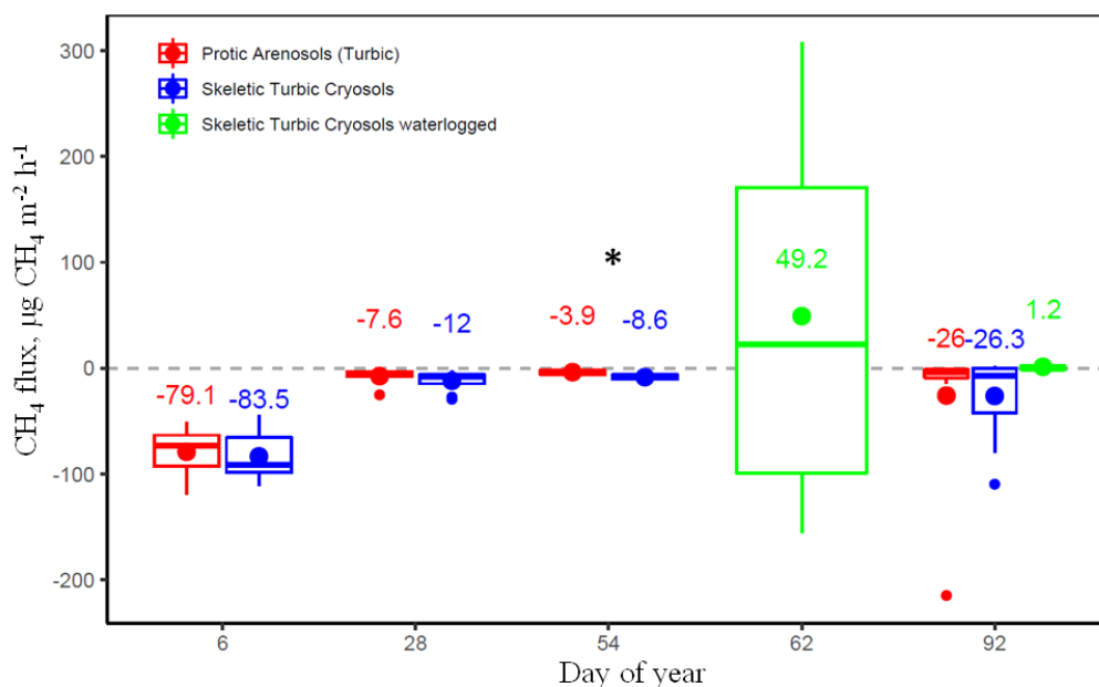
Рис. 1. Динамические изменения потоков \text{CH}_4 с поверхности автоморфных почв Protic Arenosols (Turbic), Skeletic Turbic Cryosols, и гидроморфных почв Skeletic Turbic Cryosols в январе-феврале 2022 г. и марте-апреле 2023 г. Цифры – средние значения, звездочкой показано достоверное различие между типами почв.
