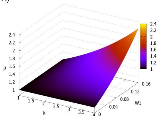
Рис.1. Коэффициент изменения глубины оттаивания грунта « \mu »: А) первый и Б) второй год после проведения снежной мелиорации при средней начальной влажности « W_1 » и различной степени увлажнения грунта деятельного слоя (« k = w_2/w_1 »)
