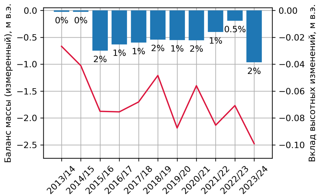
Рис. 1. Вклад изменений пространственной конфигурации ледника Альдегонда в баланс его массы. Красной линией показан измеренный баланс массы, синим цветом — вклад высотных изменений
