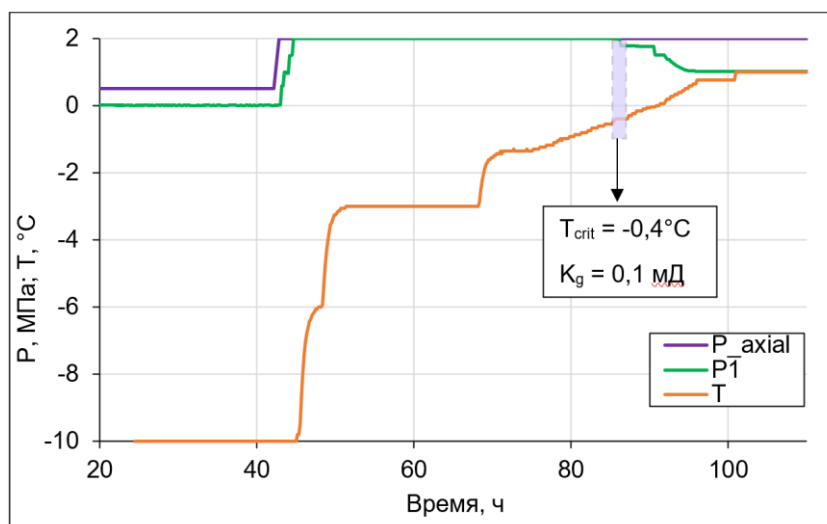
Рис. 1. Изменение термобарических условий в фильтрационном эксперименте в ходе медленного нагрева мерзлого образца суглинка. P_{axial} - осевое давление, P_1 – давление на входе в образец, T – температура.
