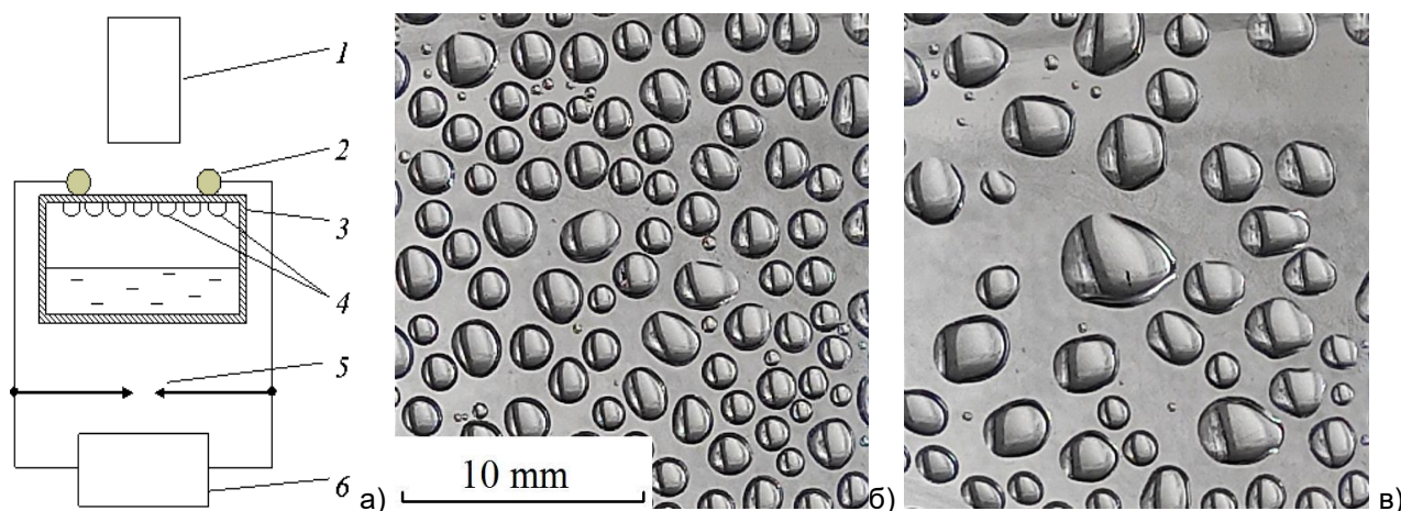
Рис. 1. Блок-схема установки. 1 – фотокамера, 2- цилиндрический электрод, 3 – пластиковый контейнер с водой, 4 – капли воды, 5 – разрядник, 6 – электростатическая машина (а). Капли воды на стенке пластиковой бутылки до приложения высокого напряжения (б), после приложения высокого напряжения (в).
