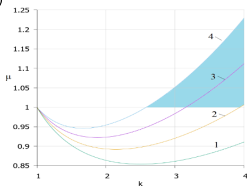
Рис.2. А) - степень изменения глубины оттаивания « \mu » на второй год после снежной мелиорации в зависимости от начальной влажности грунта « W_1 » (до проведения снежной мелиорации): 1 - W_1 = 0,1 ; 2 - W_1 = 0,12 ; 3 - W_1 = 0,14 . 4 - W_1 = 0,16 ; Б) - оптимальное значение степени увлажнения грунта деятельного слоя « k » для достижения максимального уровня снижения глубины оттаивания « \mu » на второй год.
