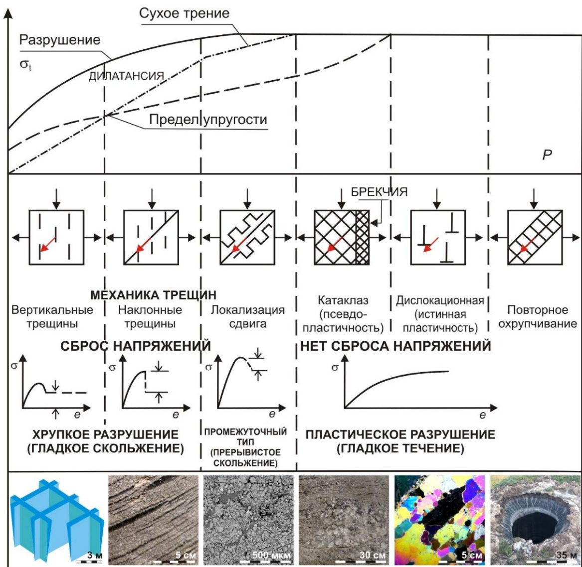
Рис. 1. Деформации мерзлых толщ по модели сплошной среды
