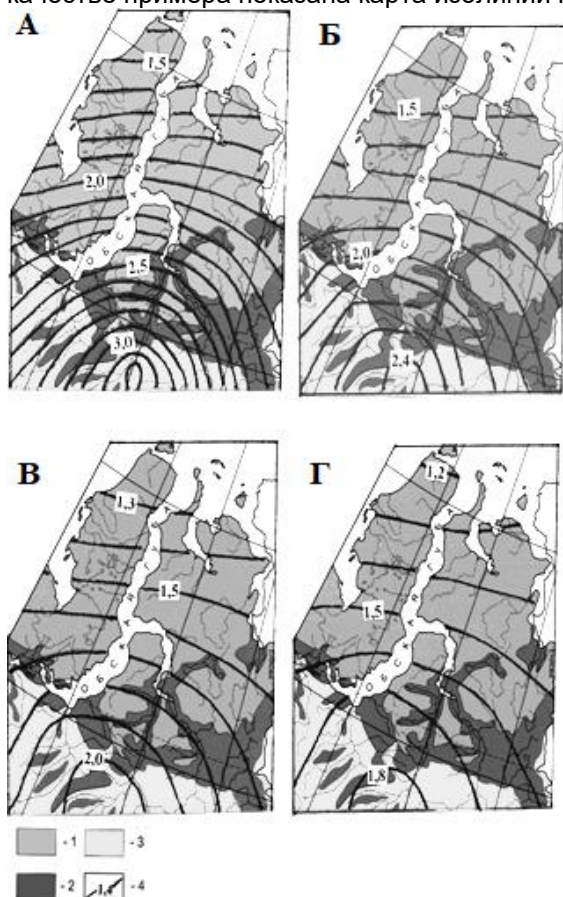
Рисунок 1. Карта изолиний k_n на территории Западной Сибири: 1 – 3 геокриологические зоны; 4 – значения коэффициента k_n ; А – при погружении свай в грунт 6 м; Б – при погружении свай в грунт 8 м; В – при погружении свай в грунт 10 м; Г – при погружении свай в грунт 12 м
