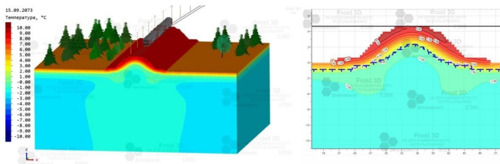
Рис.1. Пример модели железнодорожной насыпи в программном комплексе «Frost 3D» с профилем температурного поля.
