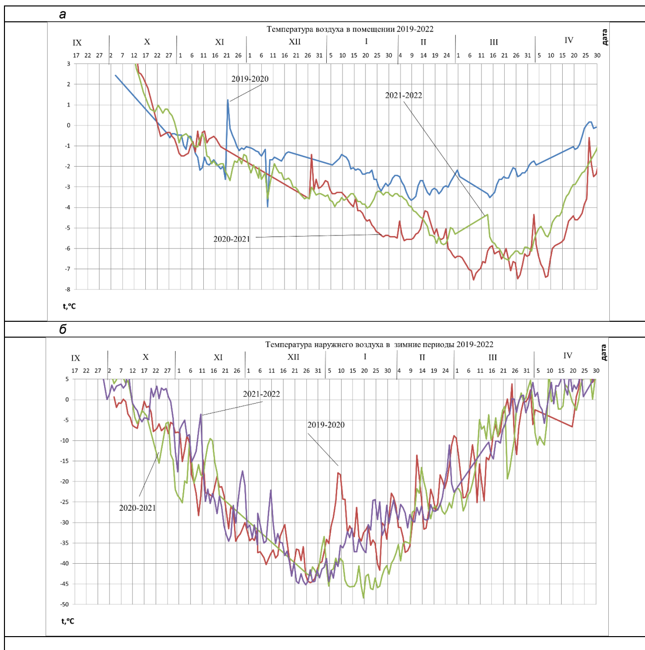
Рис. 1. Графики температур воздуха внутри (а) и снаружи (б) опытного гаража в г. Якутске при V \sim 50 \text{ м}^3 :
