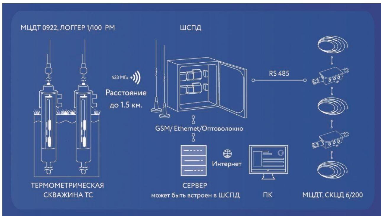
Рис.2. Конфигурация автоматизированной системы температурного мониторинга грунтов
