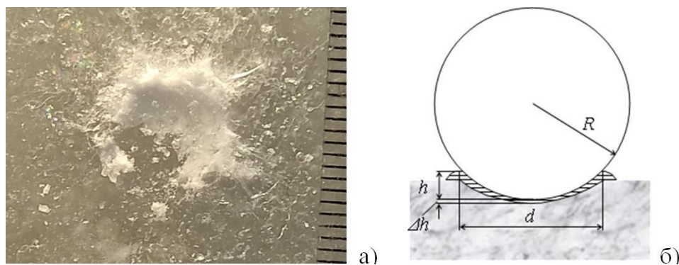
Рис. 1. Фотография лунки на фоне линейки с ценой деления 1 мм (а) и схема измерения параметров лунки (б). R – радиус шара, d – диаметр лунки, h – глубина лунки, \Delta h – толщина слоя разрушенного льда под дном лунки. Раздробленный лед показан на схеме штриховкой.
