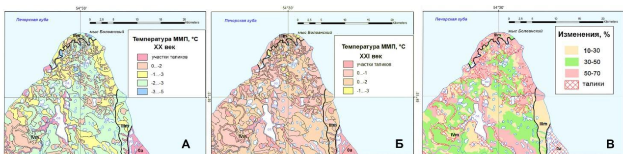
Рис. 3. Изменение среднегодовой температуры ММП для двух временных интервалов: А – 1980-е годы XX века, Б – 2020-е годы XXI века; В - относительные изменения (%) сопротивления мерзлого грунта сдвигу по поверхности смерзания с фундаментом, R_{af} , обусловленные повышением температуры ММП за 40 лет
