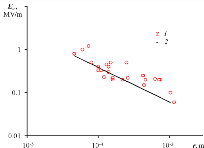
Рис. 2. Зависимость критической напряженности электрического поля E_c от среднего радиуса капель r . (1) – экспериментальные значения, (2) – теоретическая кривая.
